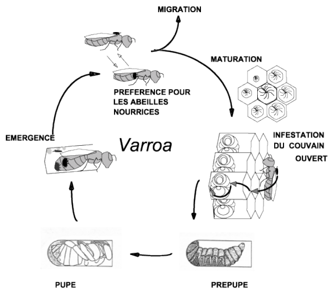
Fig. 14: Cycle de reproduction de Varroa destructor . La varroa mère et une à deux filles sortent de la cellule lors de l'émergence de l'ouvrière pour recommencer un cycle de reproduction. Quand elles infestent un faux-bourdon, 4 à 5 filles peuvent être produites. Chaque acarien peut réaliser 3 à 8 cycles de reproduction, résultant en une croissance exponentielle de la population de parasites dans la colonie.
